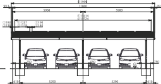
4台用(5段8列)
