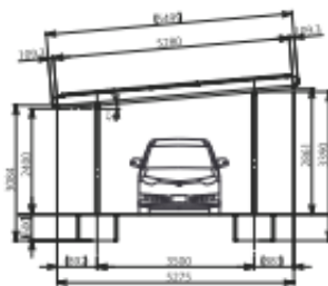
4台用(5段8列)
