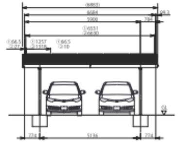
2台用(5段5列)
