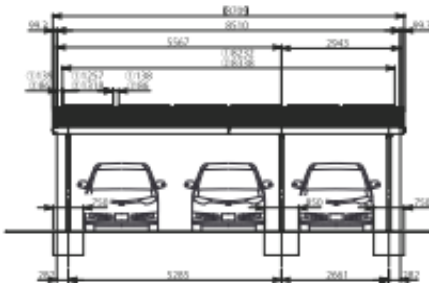
3台用(5段6列)
